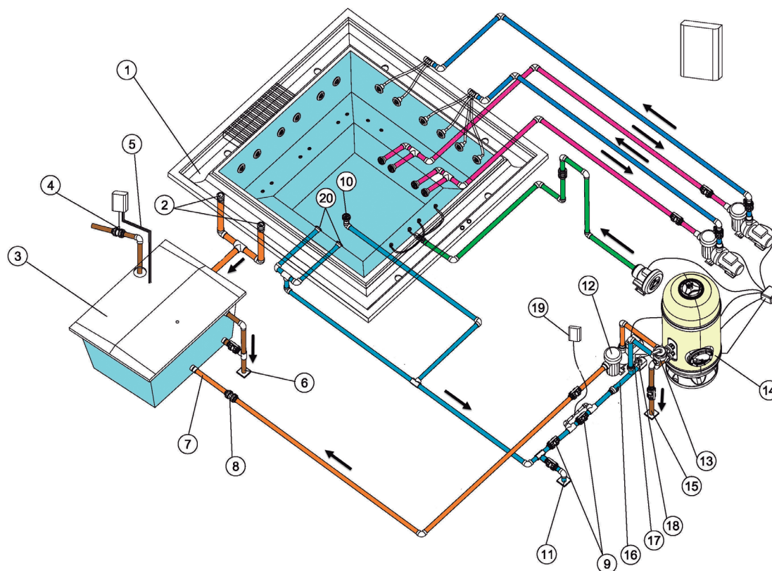
Wasserkreislaufschema des Spas mit Überlaufwanne. Option B
