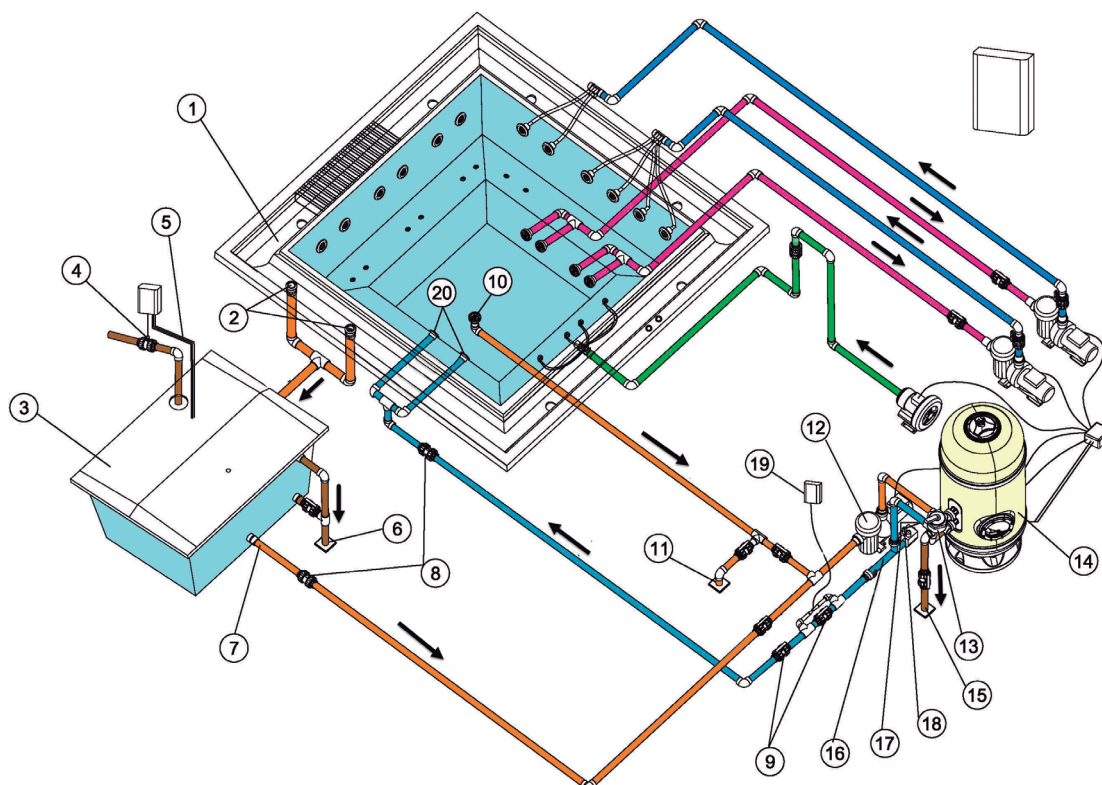
Schéma recirculation Spa à débordement. Option A.
