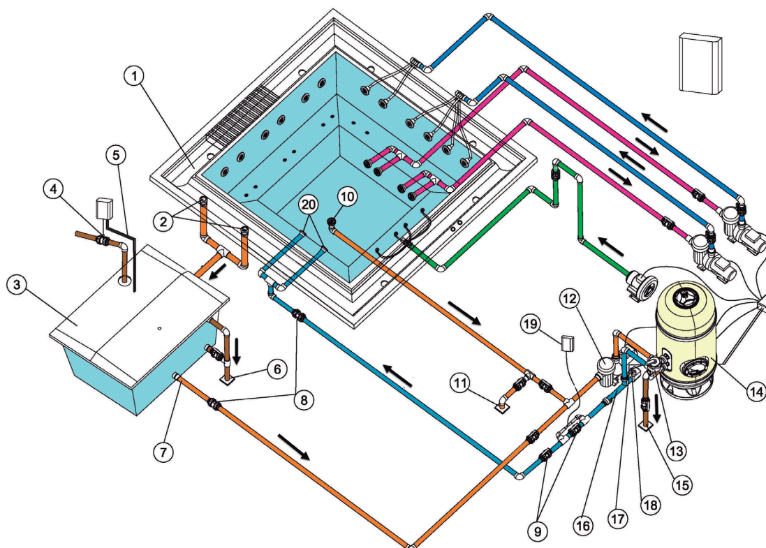
Esquema recirculação Spa com Transbordante. Opção A.
