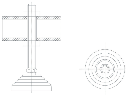
Einzeldarstellung des Regulierungstützpunkts.
