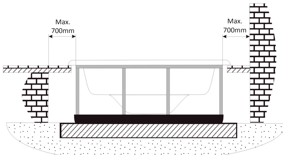
Schema Distanza minima perimetrale.
