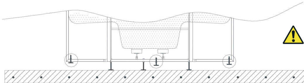
Fig. 1 Schaubild zur Höhenregulierung des Spas.
