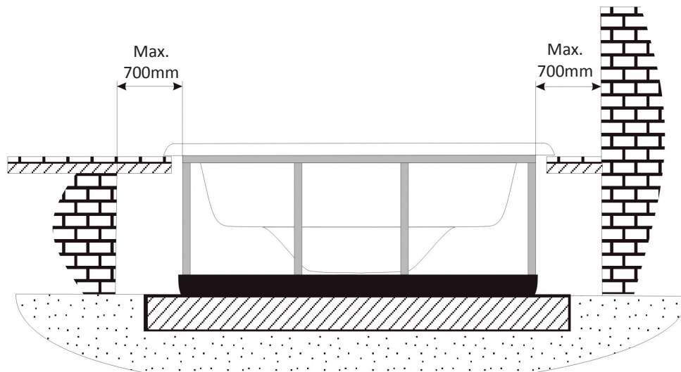
Schaubild Mindestabstand um das Spa.
