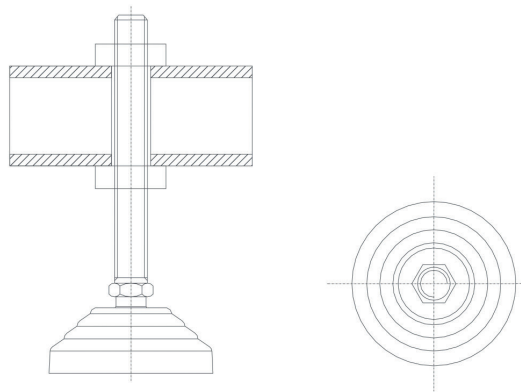
Detalle soporte de regulación.
