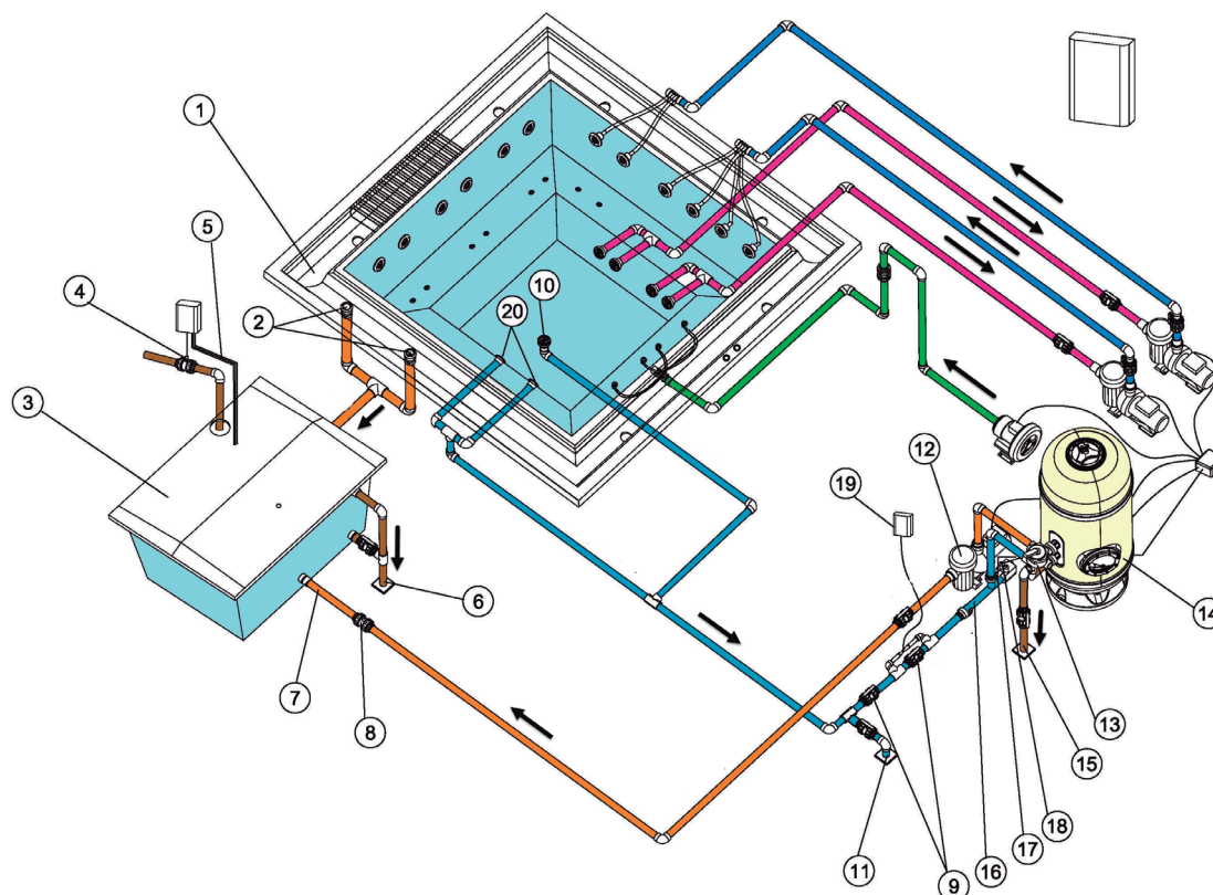
Schéma recirculation Spa à débordement. Option B.
