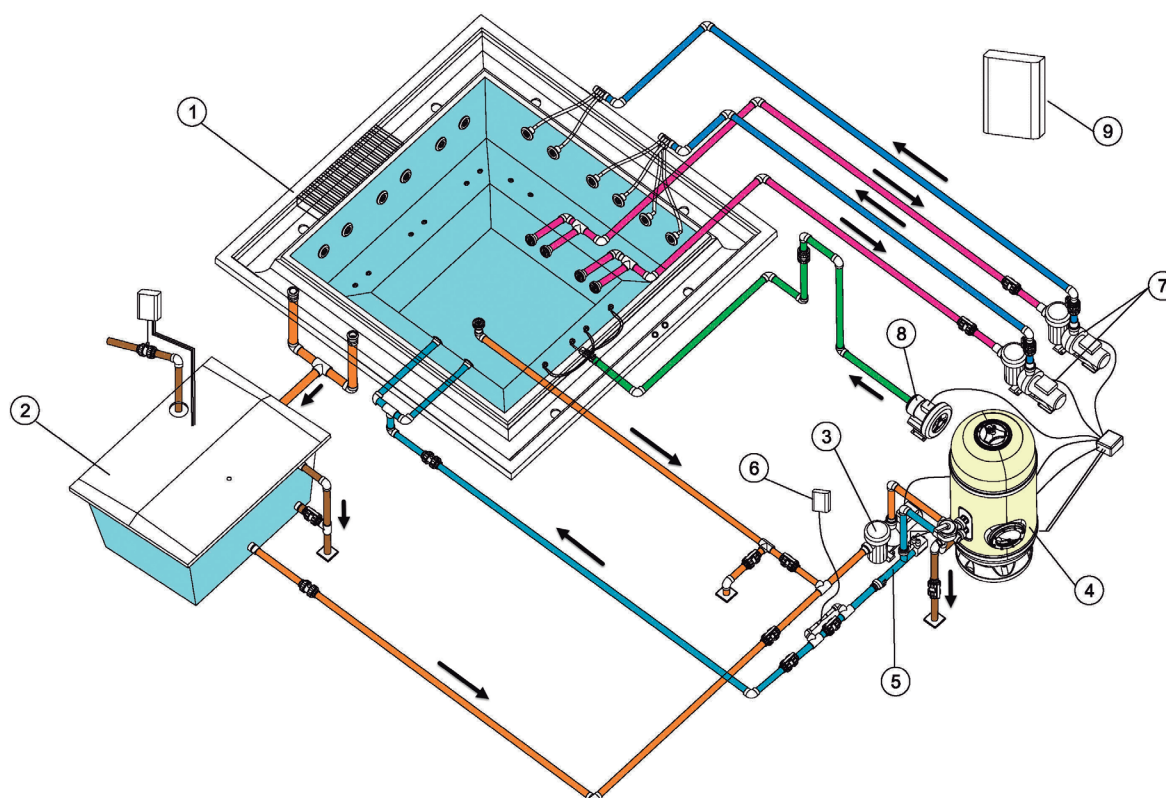
Esquema general Spa con Desbordante
