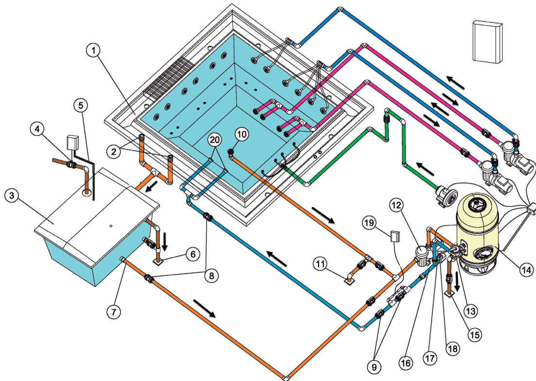
Esquema recirculación Spa con Desbordante. Opción A.
