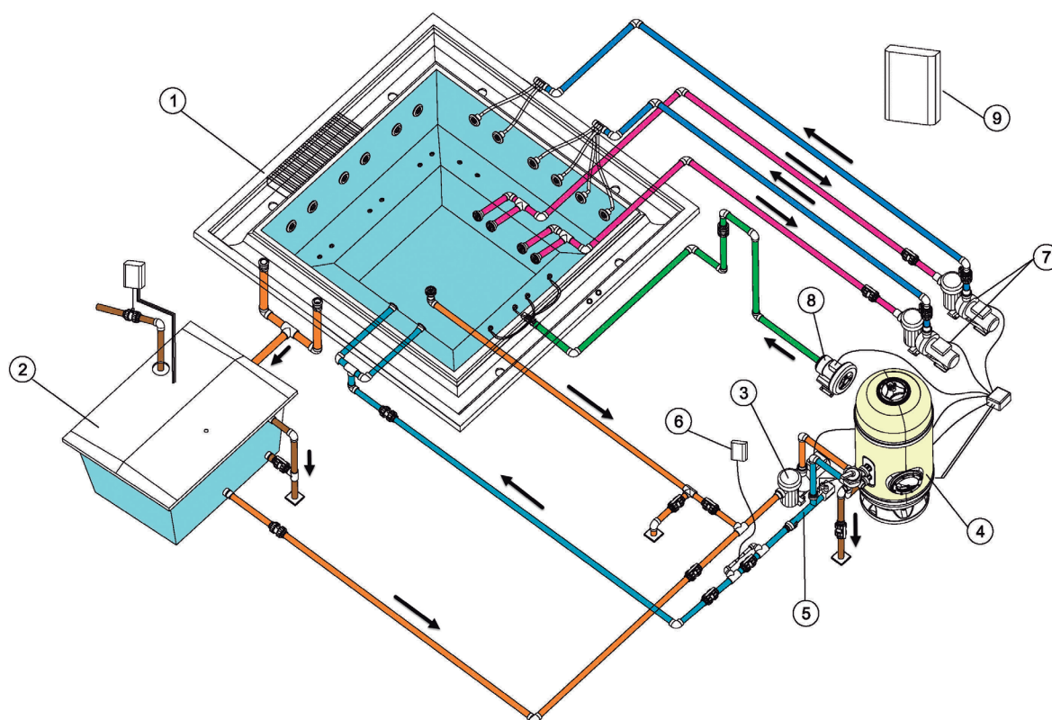
Schéma général d'un Spa à débordement.
