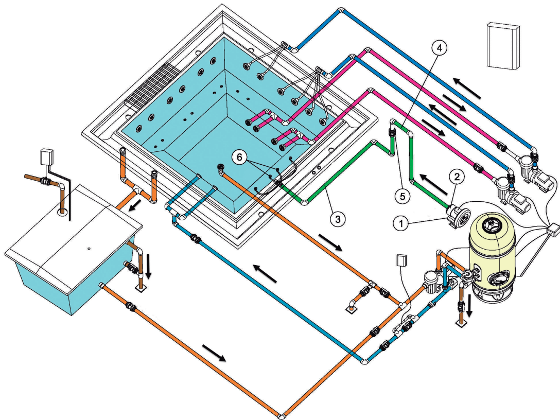
Esquema Masaje Aire Spa.
