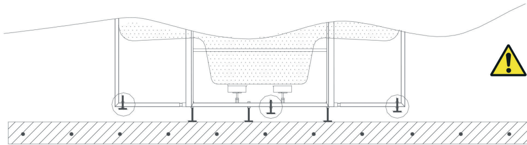
Fig. 1 Esquema regulación altura Spa.
