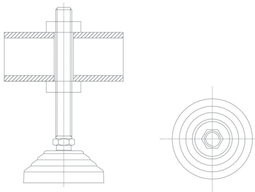
Dettaglio supporto di regolazione
