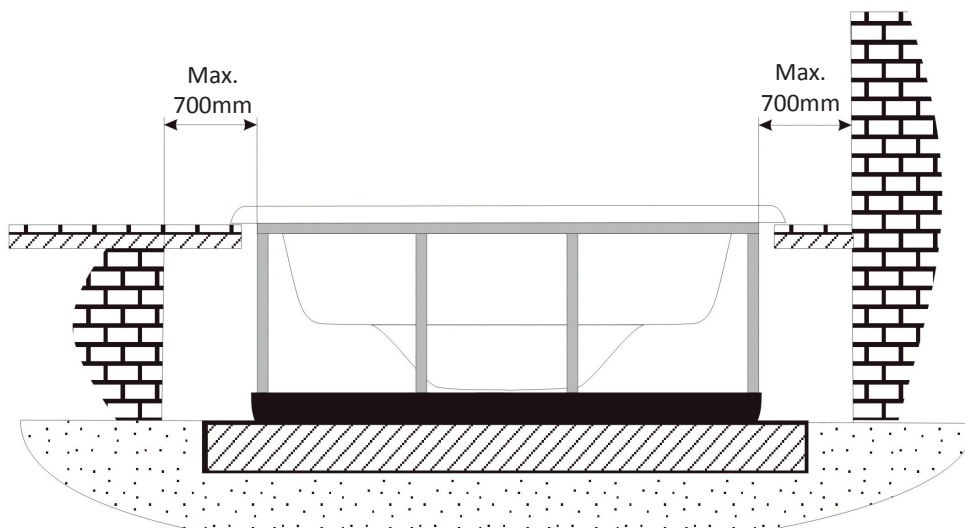
Schema minimumafstand rondom de Spa.
