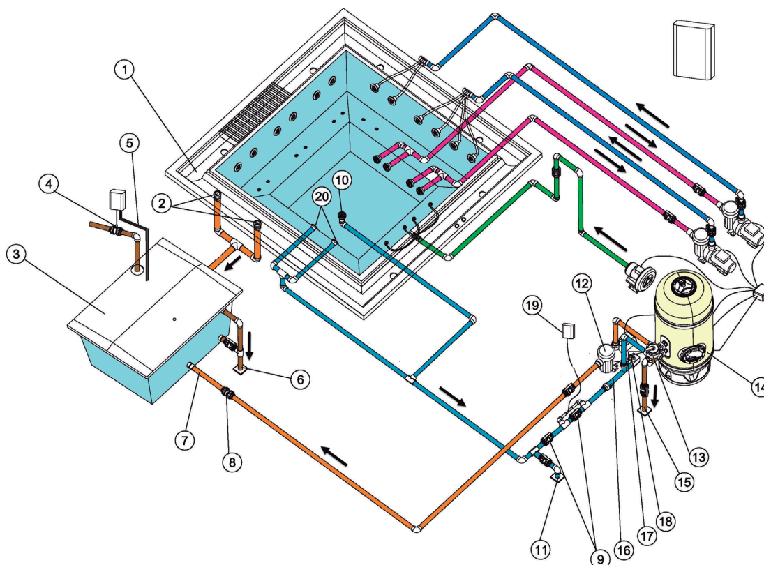
Esquema recirculación Spa con Desbordante. Opción B.
