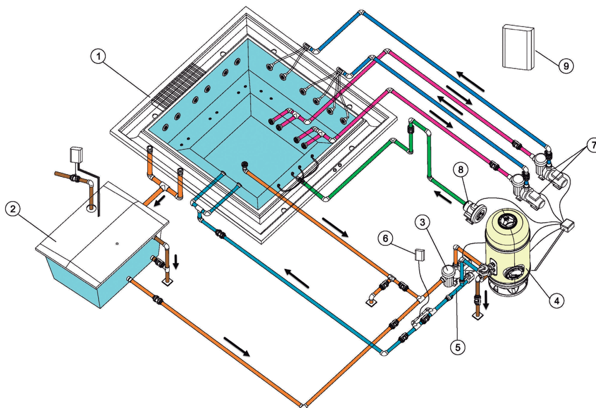
Esquema geral Spa com Transbordante.
