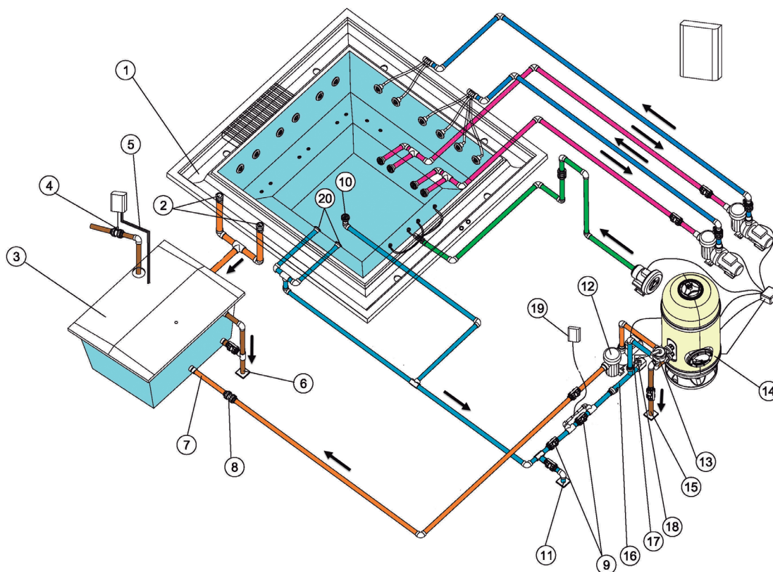
Schema recirculatie Spa met Afvloeiing. Optie B.
