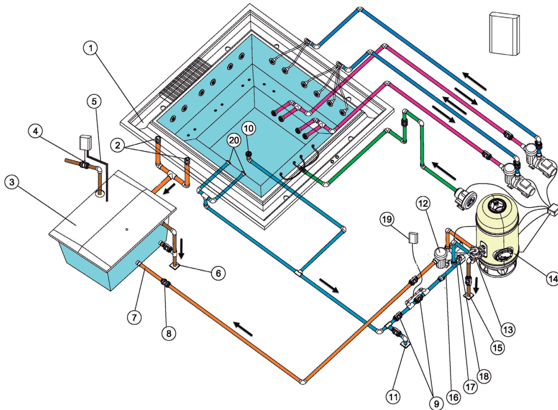
Schema di ricircolo Spa a bordo sfioratore. Opzione B.
