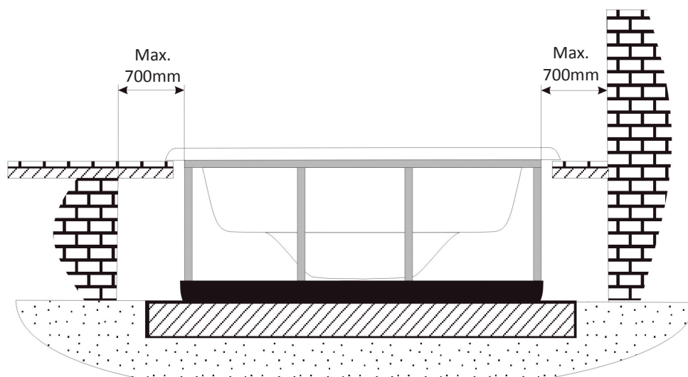
Schéma Distance minimum autour du Spa.
