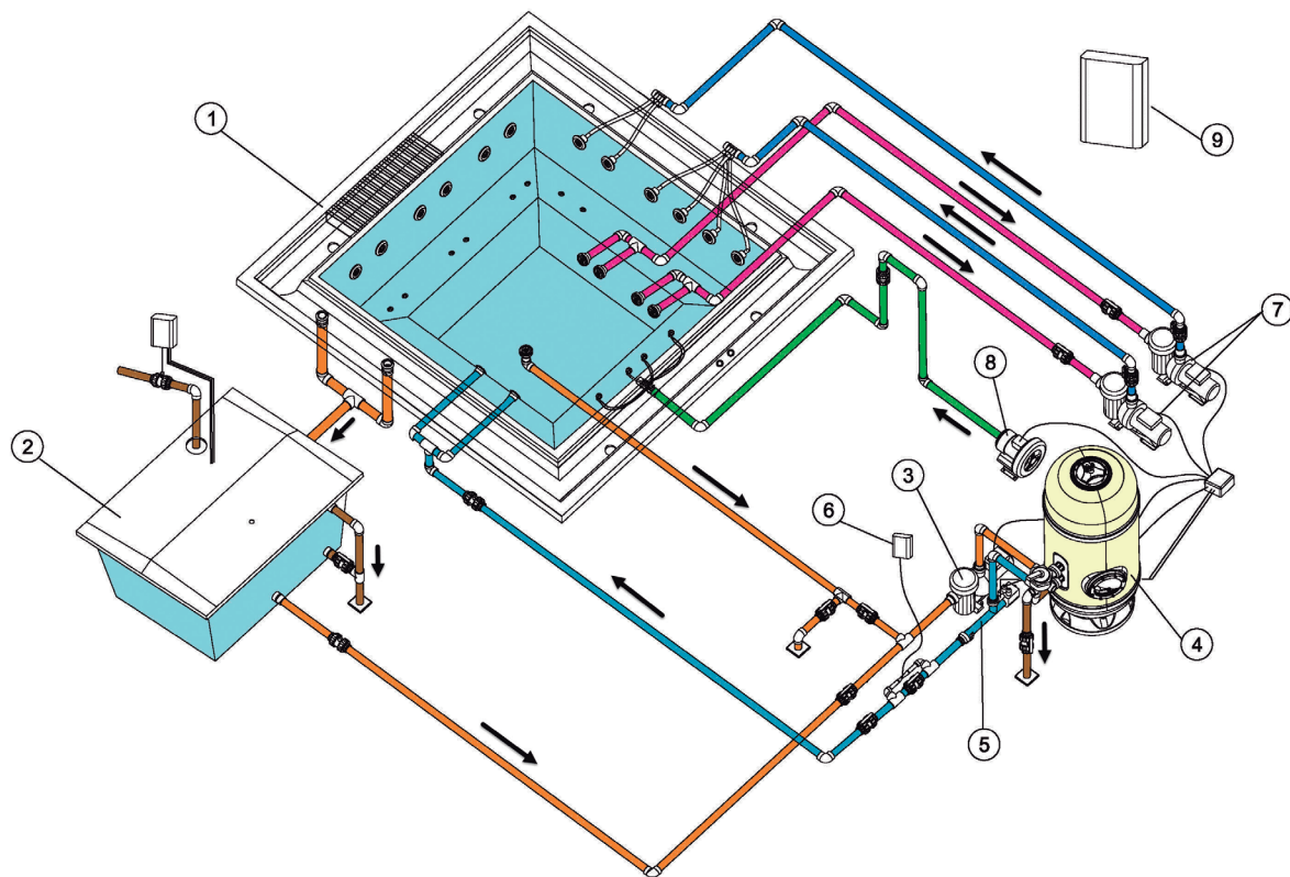
Gesamtschema des Spas mit Überlaufrinne.
