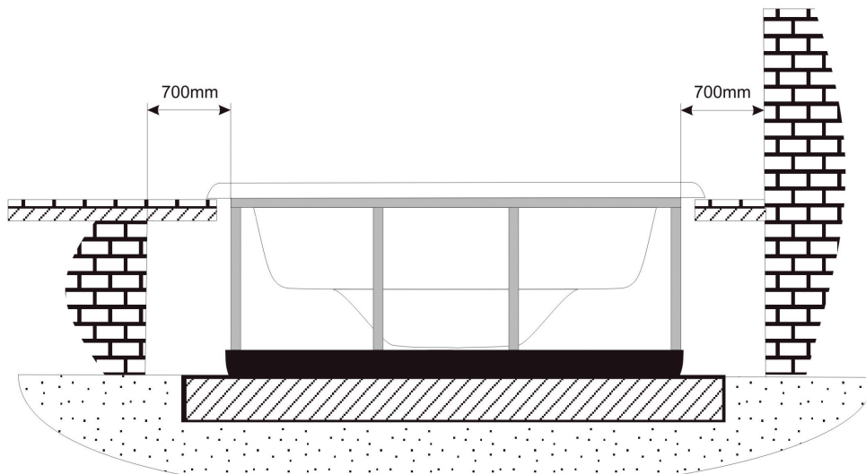
Esquema Distancia mínima alrededor del Spa
