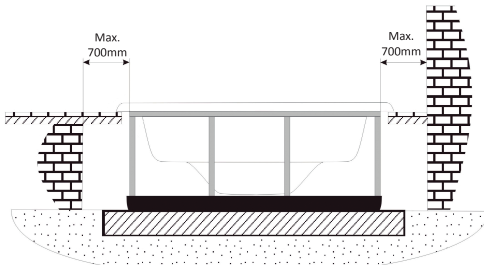
Esquema Distância mínima à volta do Spa.
